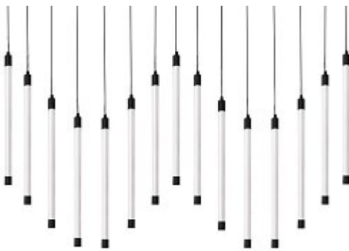
Stix array
